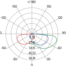
Gráfico 3 – Balizador 3W
