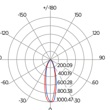
Gráfico 2 – Lâmpada PAR20 CRYSTAL 4,8W
